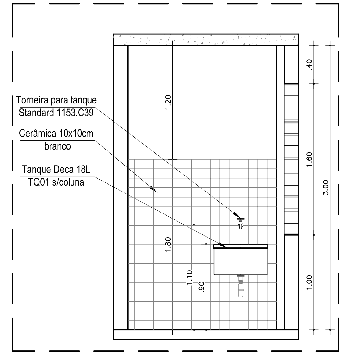
3 VISTA 2 ESC. 1:25
