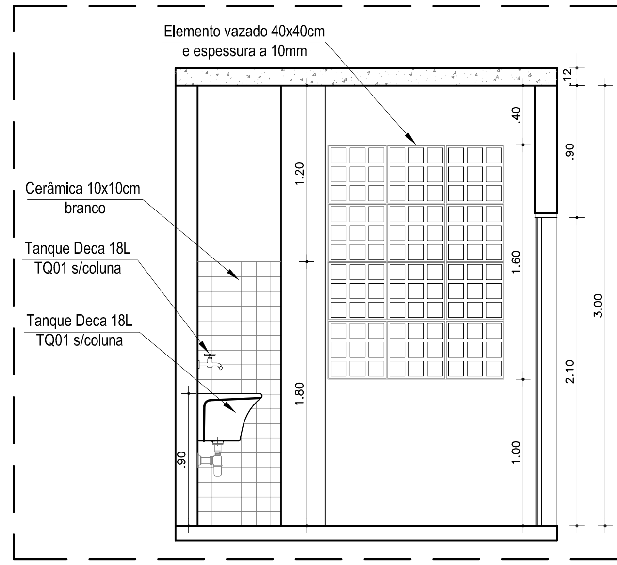
2 VISTA 1 ESC. 1:25
