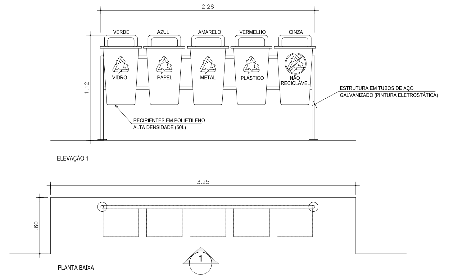
02 DET. LIXEIRA ESCALA 1/25
