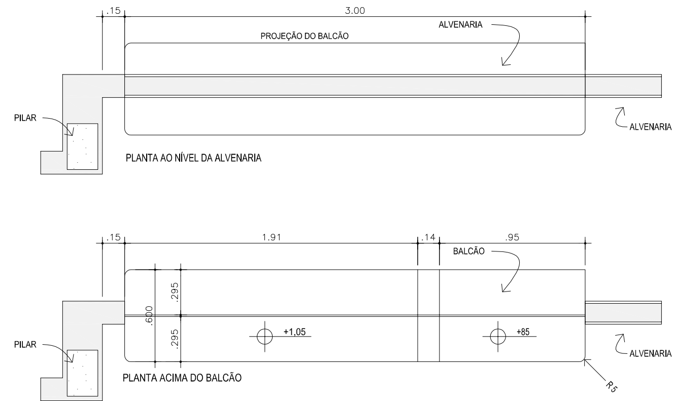
01 DET. BALCÃO RECEPÇÃO ESCALA 1/25
