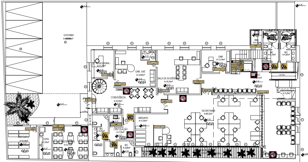
01 PLANTA BAIXA TÉRREO esc: 1/100
