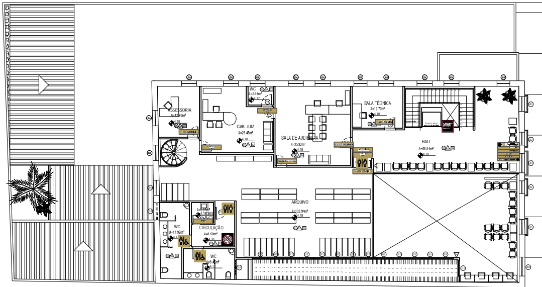
01 PLANTA BAIXA SUPERIOR esc.1/100
