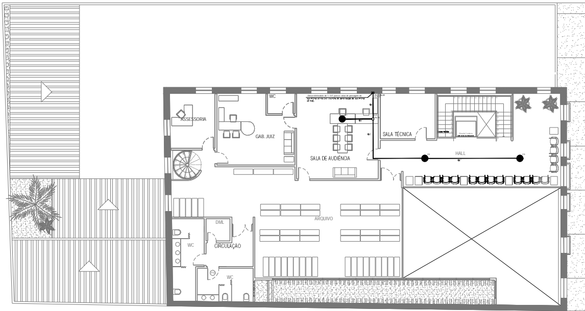
01 PLANTA BAIXA SUPERIOR ESC 1/100
