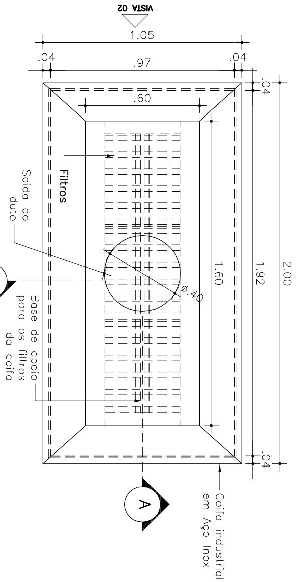
01 VISTA SUPERIOR ESCALA 1/20
