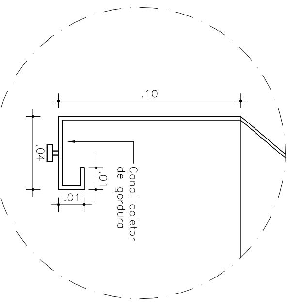
05 DETALHE 01 SEM ESCALA
