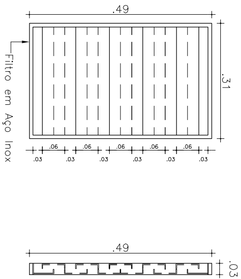
04 DETALHES DOS FILTROS ESCALA 1/10
