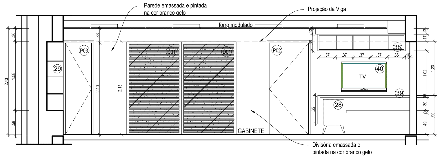
2 CORTE B esc:1/50
