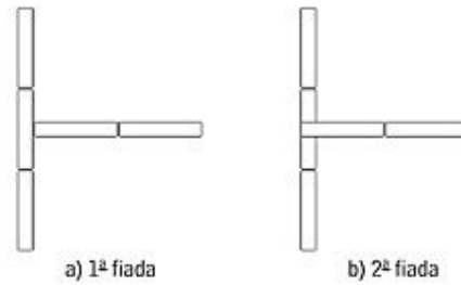
Figura 3 - Amarração de junção (T)
