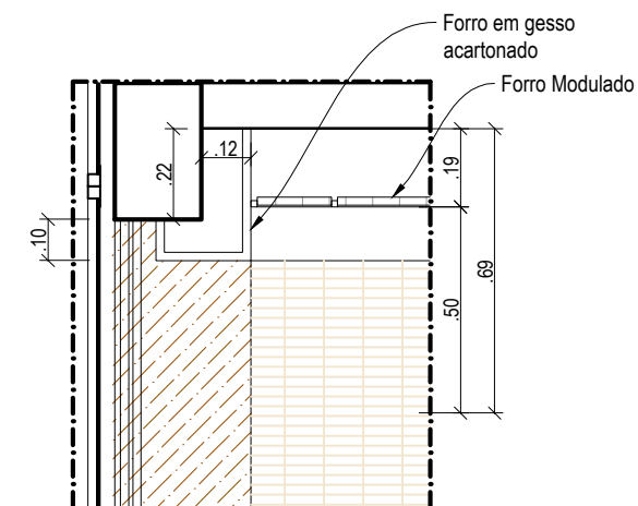
5 DETALHE 03 esc:1/20
