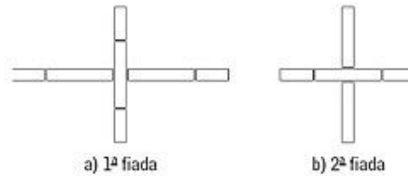
Figura 4 - Amarração em cruz
