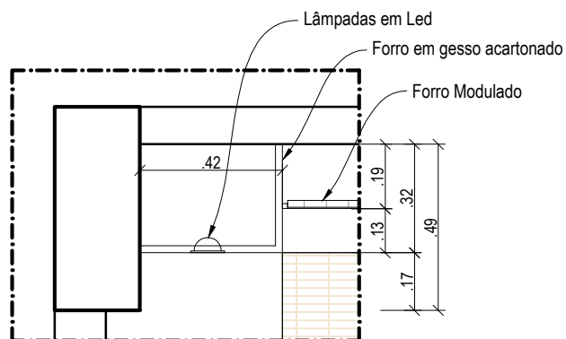
3 DETALHE 01 esc:1/20
