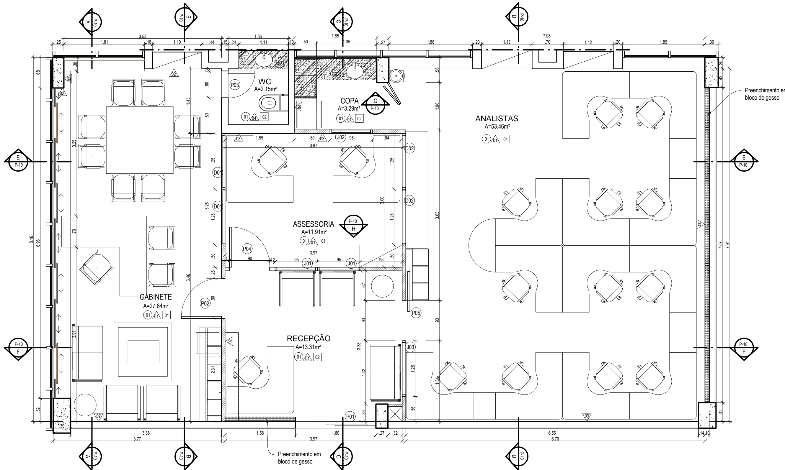
01 PLANTA BAIXA - DIVISÓRIAS E LAYOUT esc:1/50
