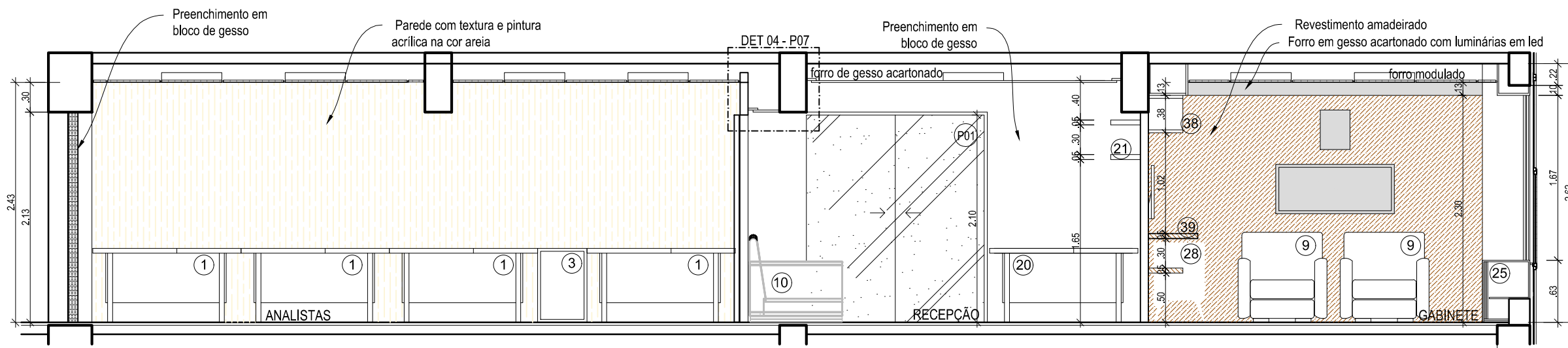
2 CORTE F esc:1/50
