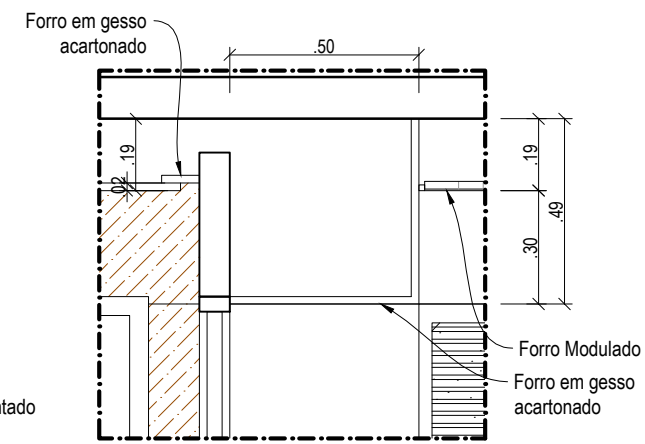
7 DETALHE 05 esc:1/20
