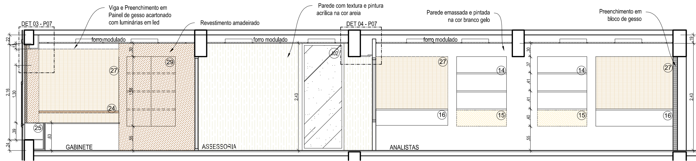
1 CORTE E esc:1/50
