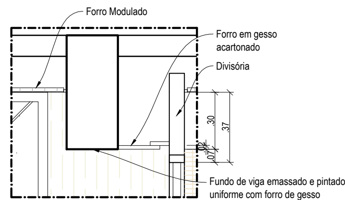
6 DETALHE 04 esc:1/20
