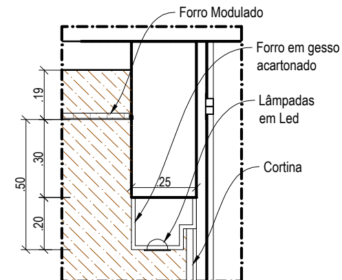
4 DETALHE 02 esc:1/20
