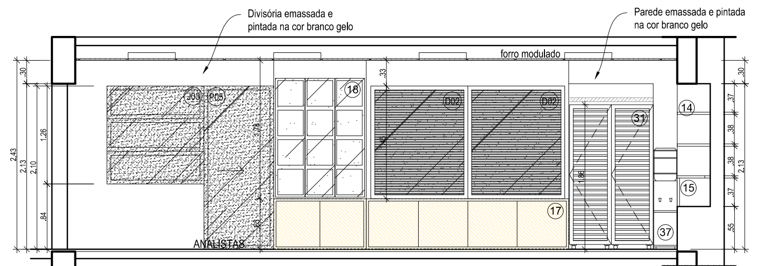
4 CORTE D esc:1/50
