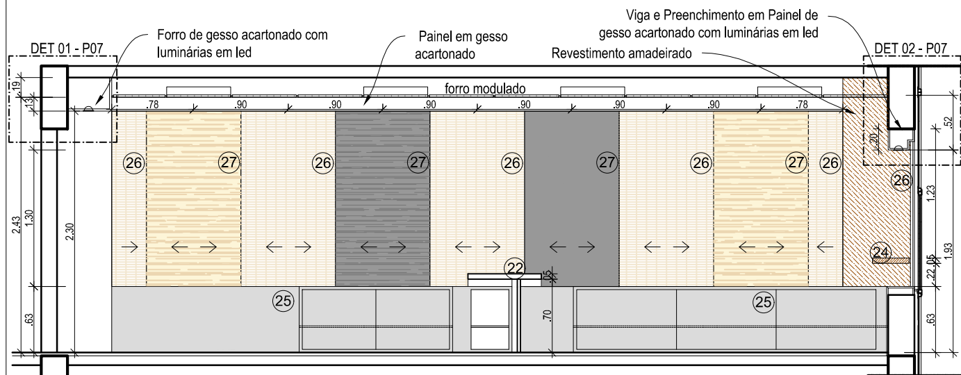
1 CORTE A esc:1/50
