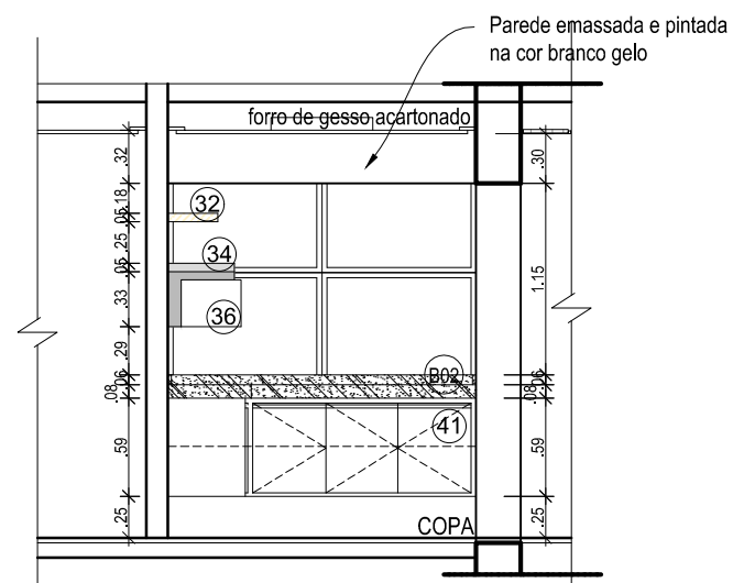
1 VISTA G esc:1/50
