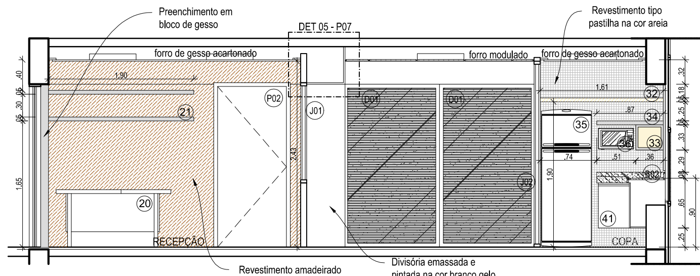
3 CORTE C esc:1/50
