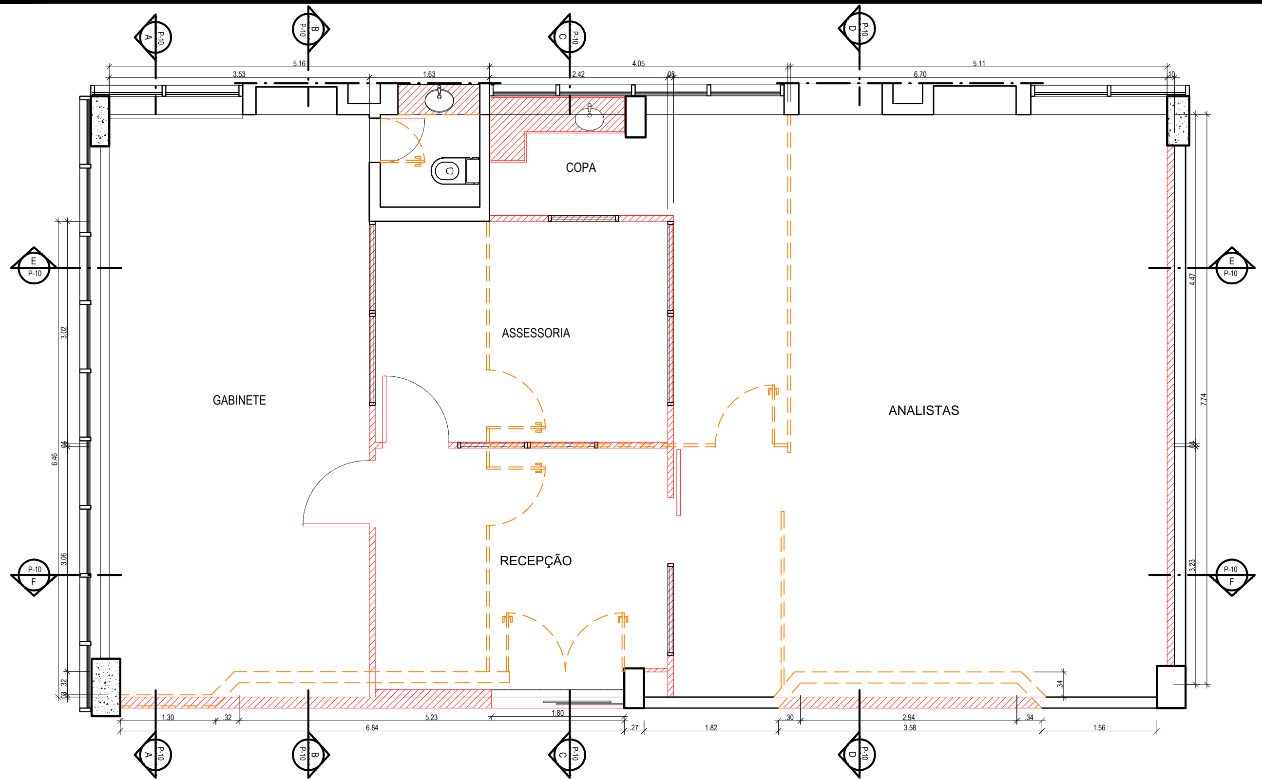
01 PLANTA BAIXA - DEMOLIR/CONSTRUIR esc:1/50
